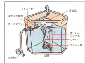
【タンク内のしくみ】
